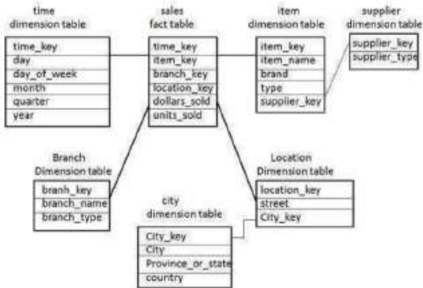
Figura 2 Modelo dimensional copo de nieve. Fuente: (Rajasekaran et al., 2020)
