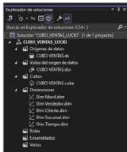
Figura 17. Creación de Cubo Dimensional.
