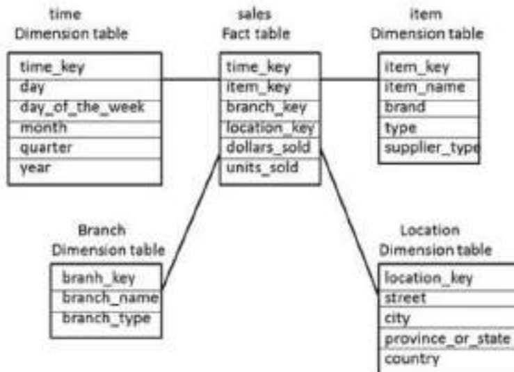
Figura 1 Modelo dimensional estrella. Fuente: (Rajasekaran et al., 2020)
