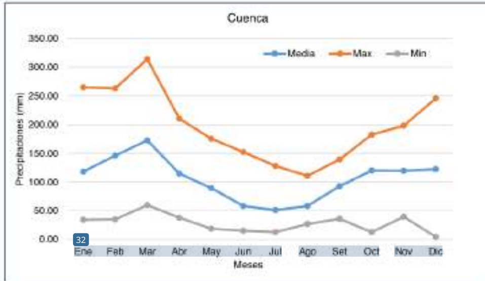
Figura 7 Curva de precipitación anual de la cuenca Rumiayacu
