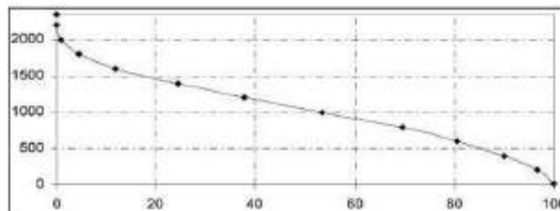
Figura 4 Representación de una curva hipsométrica
