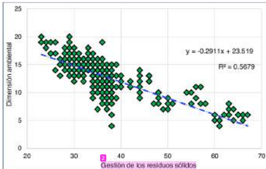
Figura 3 Gráfico de dispersión entre gestión de los residuos sólidos y la dimensión ambiental
