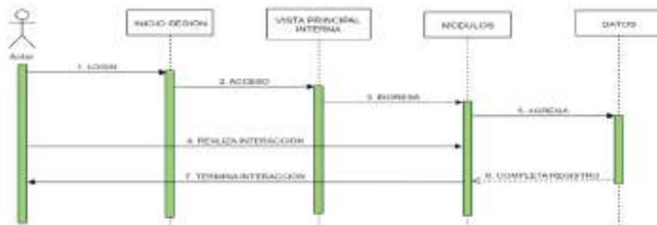
Figura 8 Diagrama de secuencias
