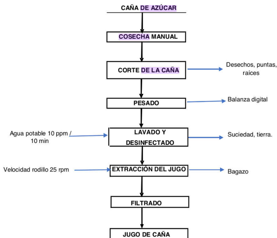
Figura 6 1 Flujograma para la obtención del jugo de caña de azúcar
