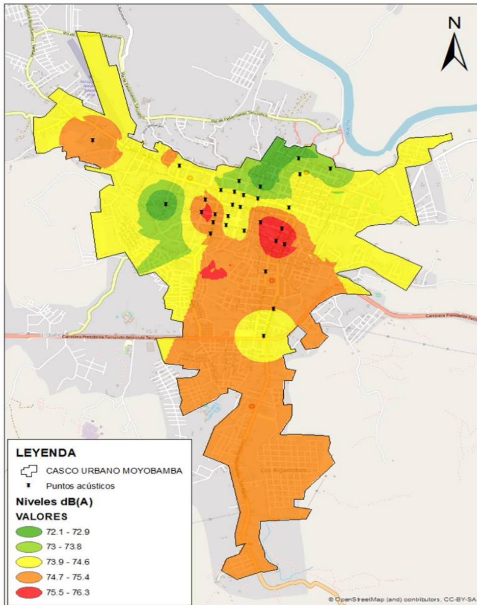
Figura 23. Mapa de ruido ciudad de Moyobamba, turno tarde.
