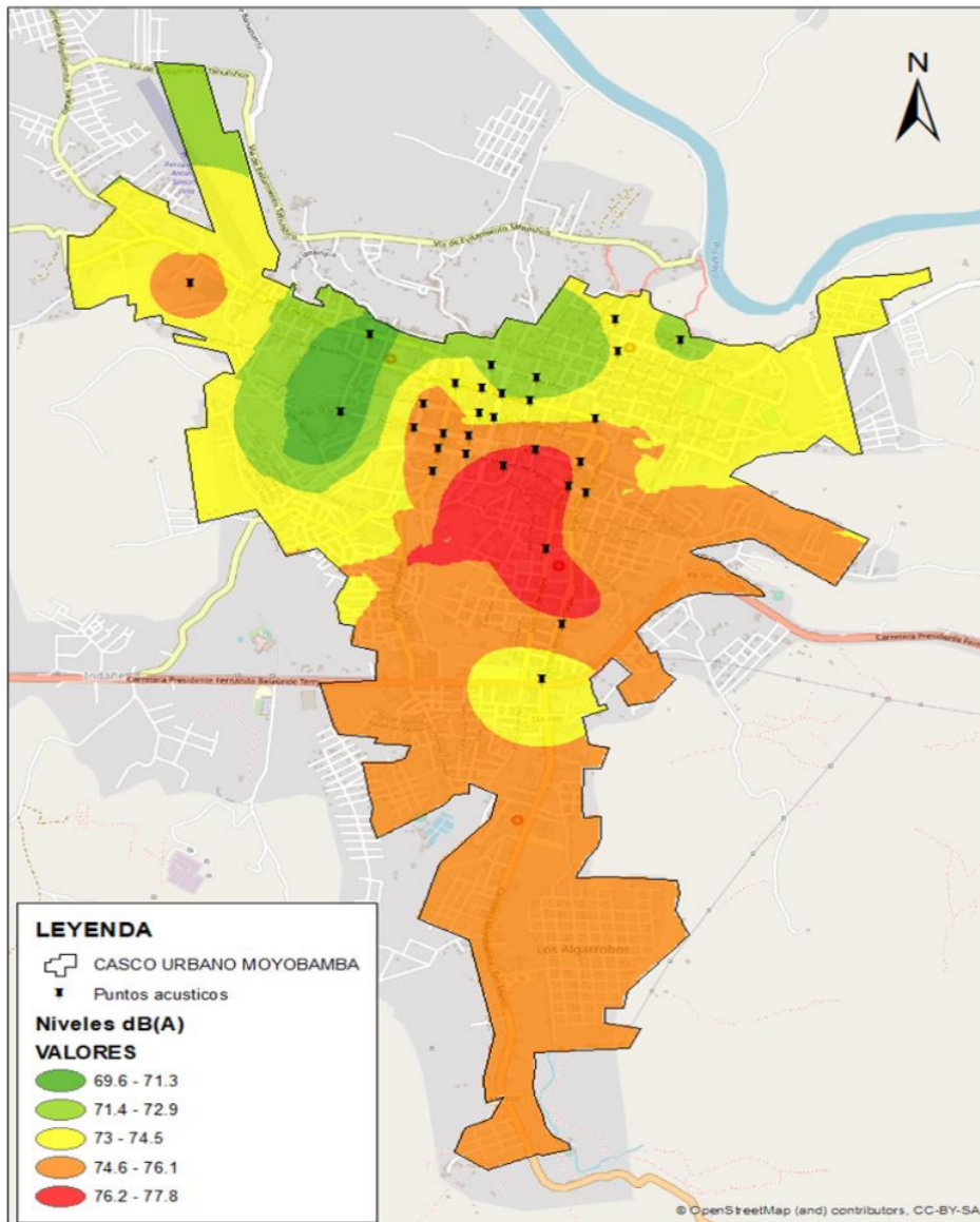
Figura 22. Mapa de ruido ciudad de Moyobamba, turno mañana.
