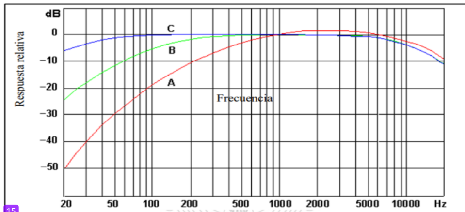
Figura 1. Curvas de ponderación A, B y C.
