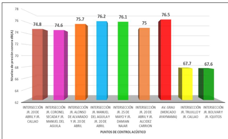
Figura 27. Resultados del nivel de presión sonora dB(A) del horario nocturno.
