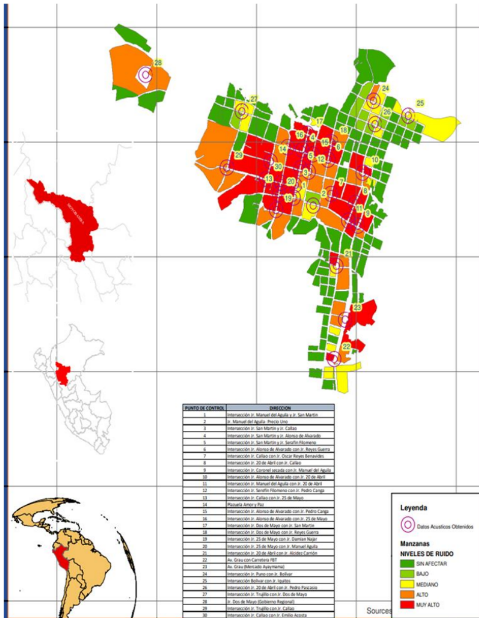
Figura 30. Mapa de ruido obtenido con opeNoise.
