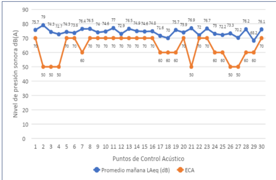
Figura 19. 27 Comparación del nivel de presión sonora del horario de la mañana.
