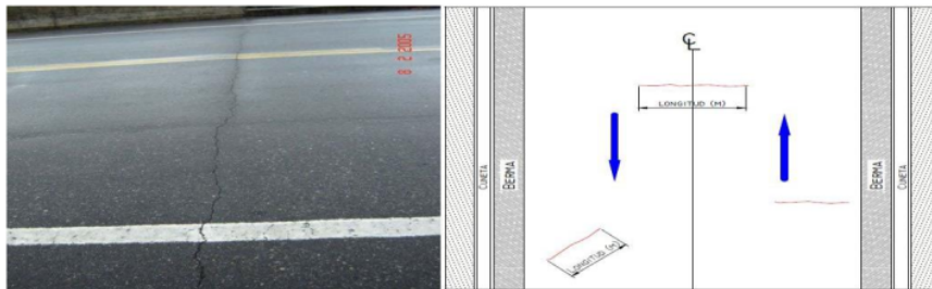
Figura 3: Fisura transversal (FT, unidad de medida: m). Discontinuidades en la carpeta Fuente: Manual MTRC, (2006, pág. 1).
