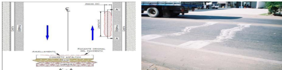
Figura 8: Ahuellamiento (AHU). Unidad de medida: m^2 Fuente: Manual MTRC (2006, pág. 13)
