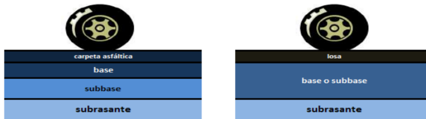
Figura 2: Esquema del paquete estructural para pavimento flexible y rígido Fuente: (Rodríguez, 2009, pág. 5)
