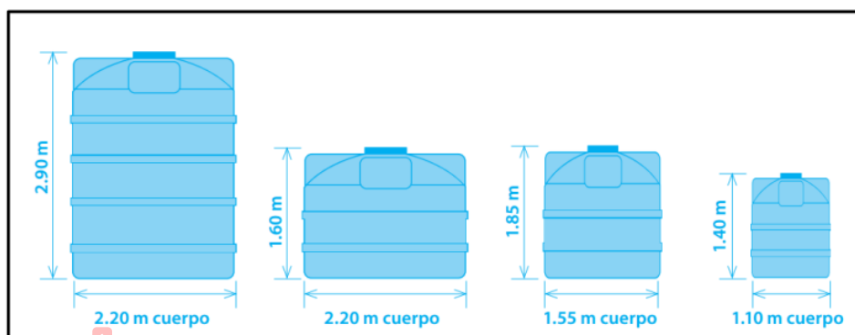
Figura 4. Dimensiones de un Tanque Cisterna Marca Rotoplas.
