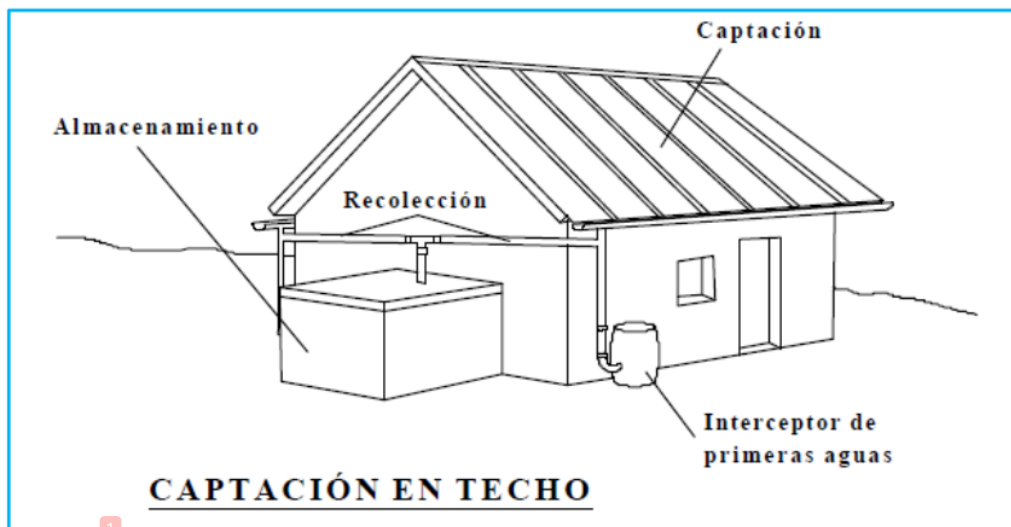
Figura 2. Esquema de un sistema de Aprovechamiento de Aguas Pluviales.
