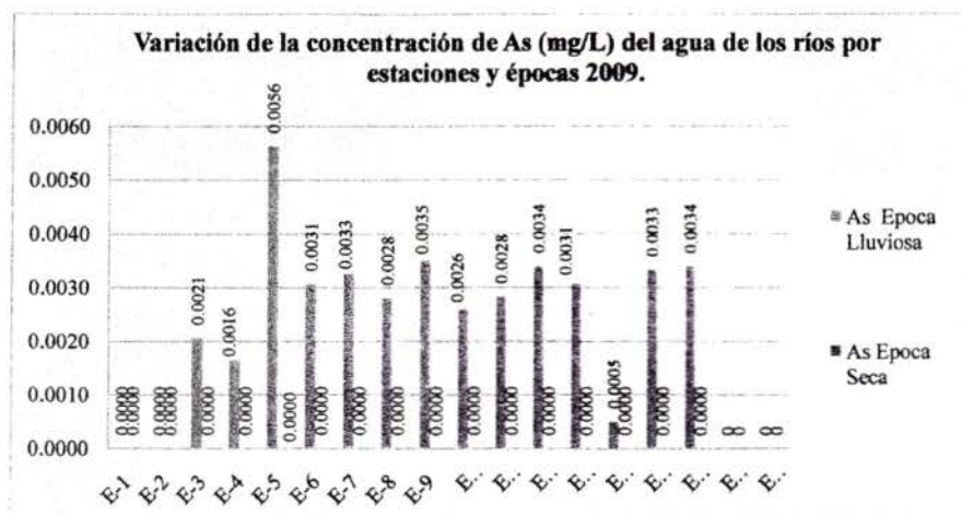
Gráfico N° 07: Variación de la concentración de As (mg/l) en el agua de los ríos evaluados por estaciones y por épocas. 2009
