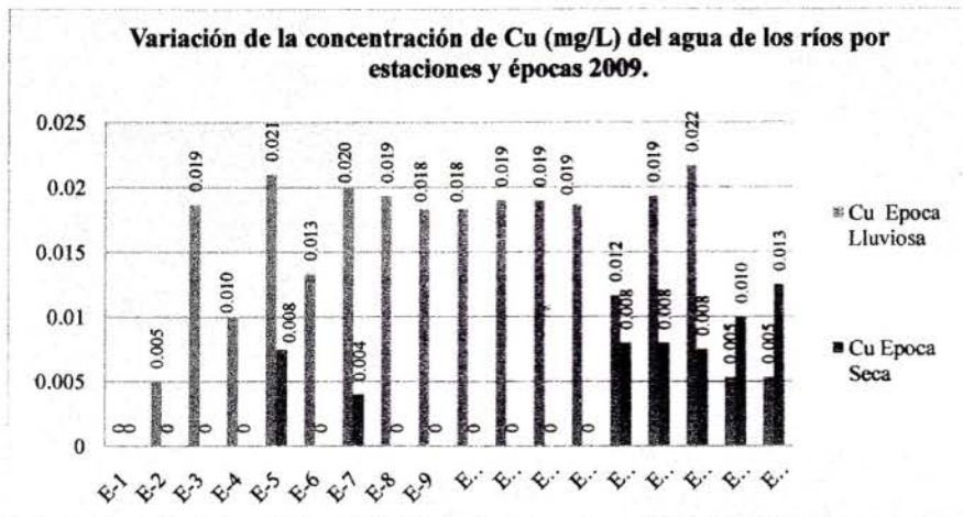
Gráfico N° 08: Variación de la concentración de Cu (mg/L) en el agua de los ríos evaluados por estaciones en época lluviosa y seca. 2009
