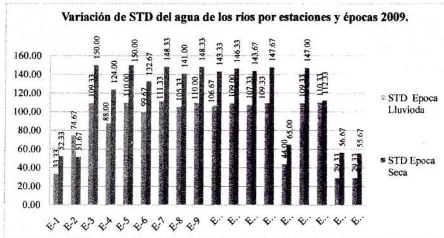
Gráfico N° 03: Variaciones de sólidos totales disueltos en el agua de los ríos evaluados por estaciones en época lluviosa y seca 2009.
