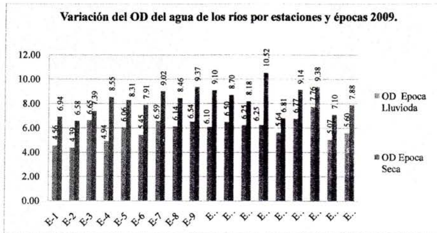
Gráfico N° 04: Variaciones de oxígeno disuelto en el agua de los ríos evaluados por estaciones en época lluviosa y seca.2009
