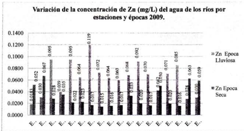
Grafico N° 13: Variación de la concentración de Zn (mg/L) en el agua de los ríos evaluados por estaciones y por épocas. 2009
