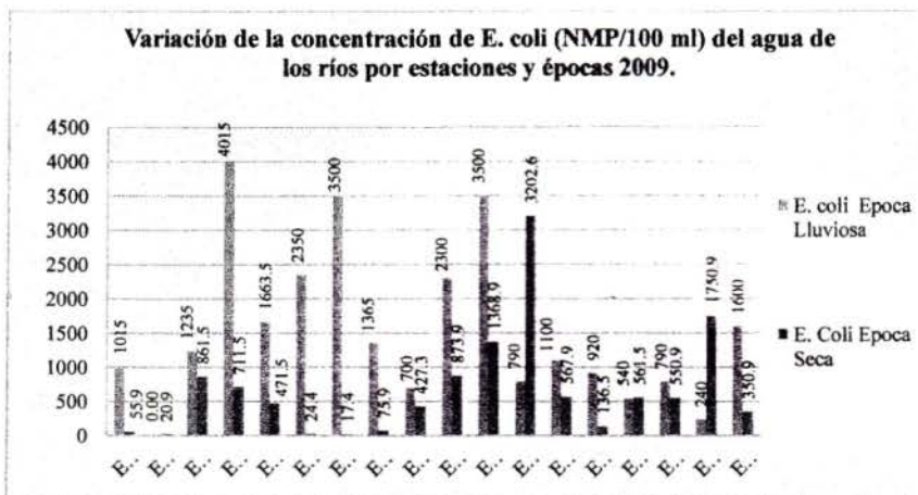
Gráfico N° 16: Variación de la concentración de E. Coli (NMP/100ml) presente en el agua de los ríos en época lluviosa y época seca. 2009
