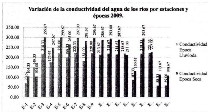
Grafico N°05: Variación de la conductividad del agua de los ríos evaluados por estaciones en época lluviosa y seca.2009
