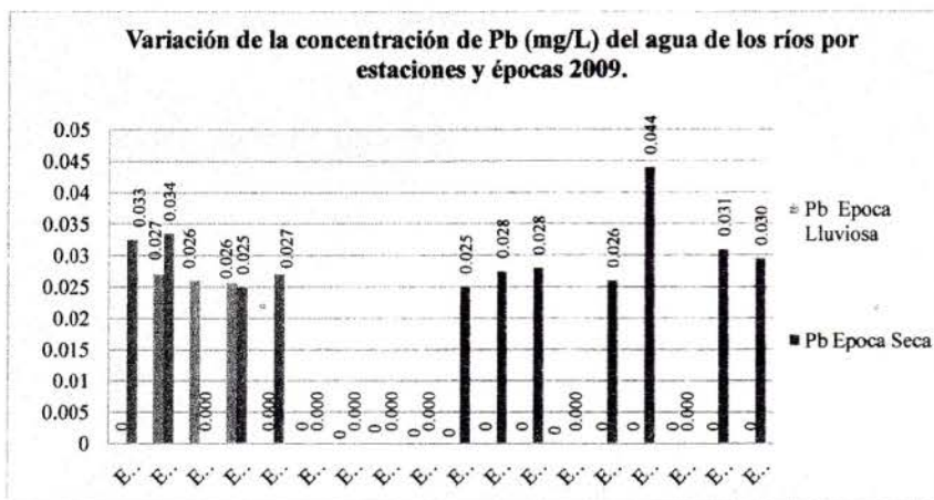
Grafico N° 12: Variación de la concentración de Pb (mg/L) en el agua de los ríos evaluados por estaciones y por épocas. 2009
