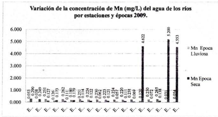
Grafico N° 11: Variación de la concentración de Mn (mg/L) en el agua de los ríos evaluados por estaciones y por épocas. 2009
