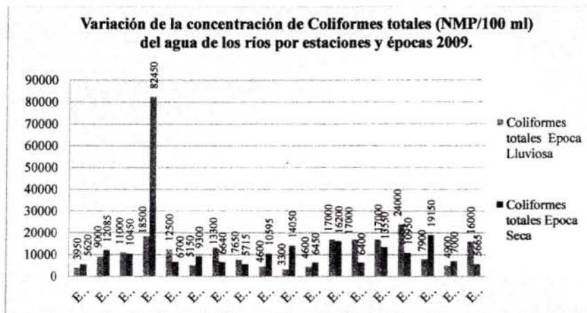
Gráfico N° 14: Variación de la concentración de Coliformes totales (NMP/100ml) presentes en el agua de los ríos evaluados en época lluviosa y época seca. 2009
