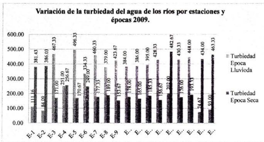
Grafico N° 06: Variación de la turbiedad del agua de los ríos evaluados por estaciones en época lluviosa y seca 2009.
