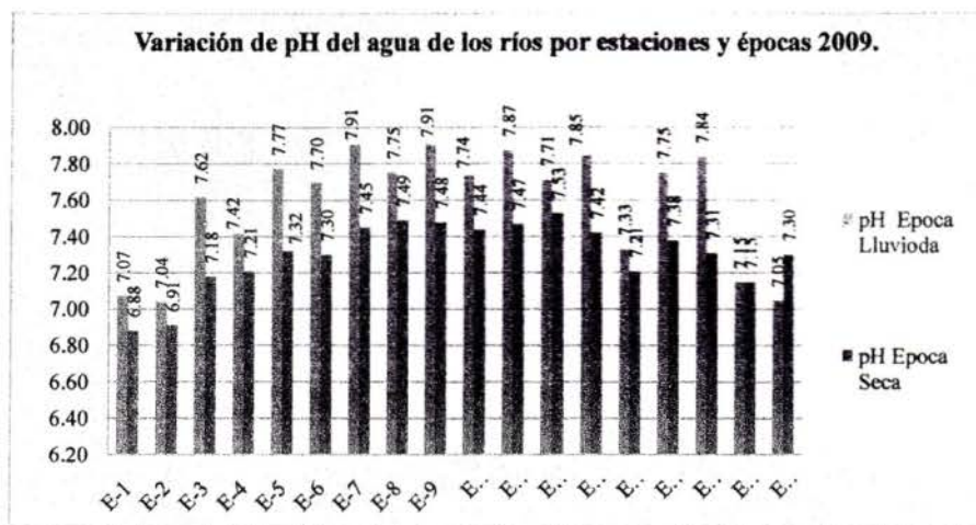
Grafico N° 02: Variación del pH del agua de los ríos evaluados por estaciones en época lluviosa y seca 2009.
