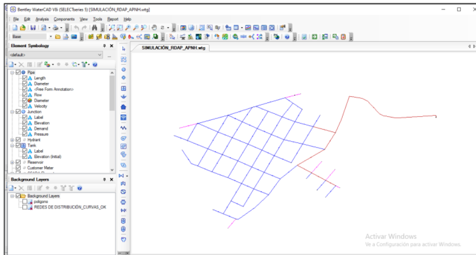
Figura 10. Red de distribución importada al Watercad
