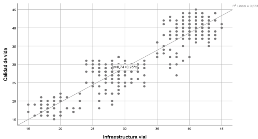
1 Figura 1. Gráfico de dispersión de los datos de la muestra de la investigación
