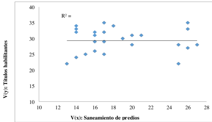
Figura 3. Diagrama de dispersión de las variables estudiadas.
