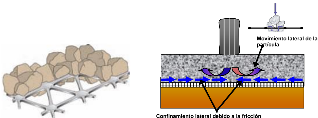
Figura 13. Confinamiento lateral e incremento del módulo (Fuente: Use of Geogrids in Pavement Construction. USACOE ETL 1110-1-189)
