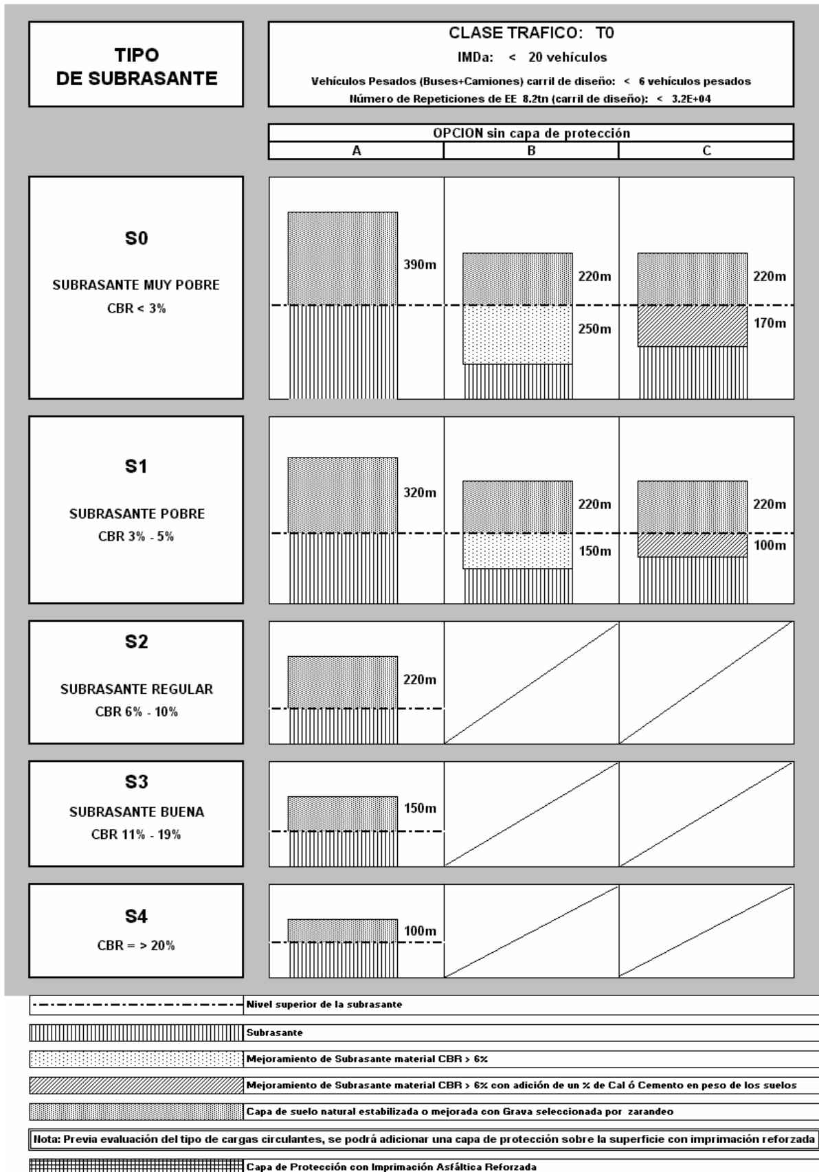
Figura 9. Catálogo de estructuras de pavimento. (Fuente: Manual para el Diseño de Carreteras No Pavimentadas de Bajo Volumen de Tránsito.)
