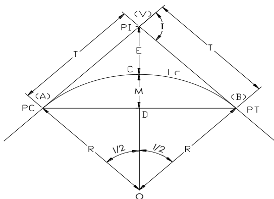
Figura 4. Elementos de una Curva Simple (Fuente: Manual para el Diseño de Carreteras no Pavimentadas de Bajo Volumen de Tránsito).
