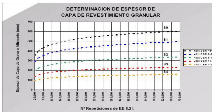
Figura 8. Determinación de espesor de capa de revestimiento granular. (Fuente: Manual para el Diseño de Carreteras No Pavimentadas de Bajo Volumen de Tránsito.)
